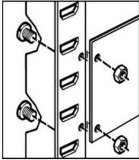
SĀNU DISTANCES STIPRINĀŠANA
