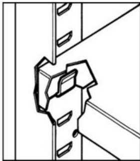
PLAUKTU PLĀTNES BALSTĀS UZ NESOŠAJIEM ĀĶIEM
