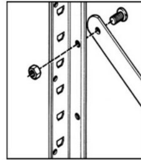
AIZMUGURES KRUSTA STIPRINĀŠANA (stiprina parasti katrai otrai sekcijai)
